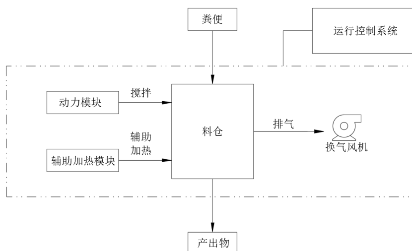
图1 船上生活污水（粪便类）生物处理装置组成示意图
